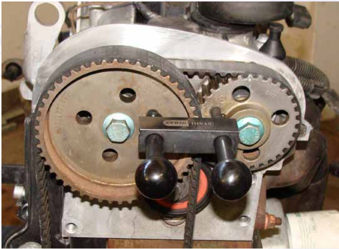
NOCKENWELLENFIXIERUNG
