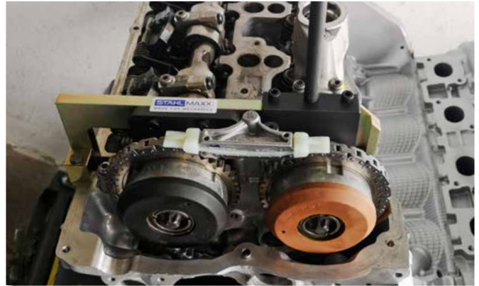
EINSTELLEHRE FÜR NOCKENWELLEN
